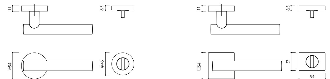
Measurements for Hotel Entrance Rose & Thumb Turn プレート・サムターンの寸法図
